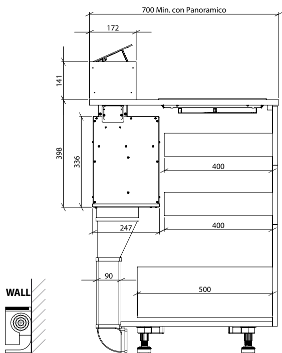
Motore in posizione anteriore (installazione a parete) Motor in front position (wall installation)
