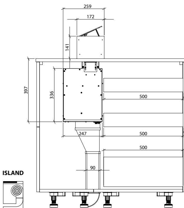
Motore in posizione posteriore (installazione ad isola) Motor in rear position (island installation)
